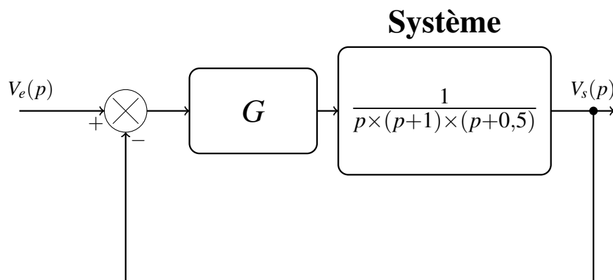
FIGURE 1 – Système étudié
